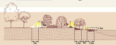
MẶT CẮT CHIẾU SÁNG BỜ HỒ VÀ ĐƯỜNG DẠO
